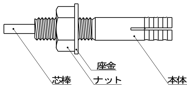
ハイアンカー DC タイプの部品構成
