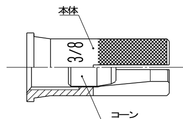
ハイアンカーTNW3030 の 部品構成
